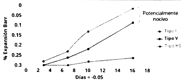
EXPANSIÓN PROVOCADA POR LA REACCIÓN ALCALÍ - AGREGADO
